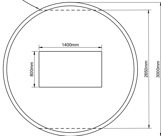
LID PLAN
